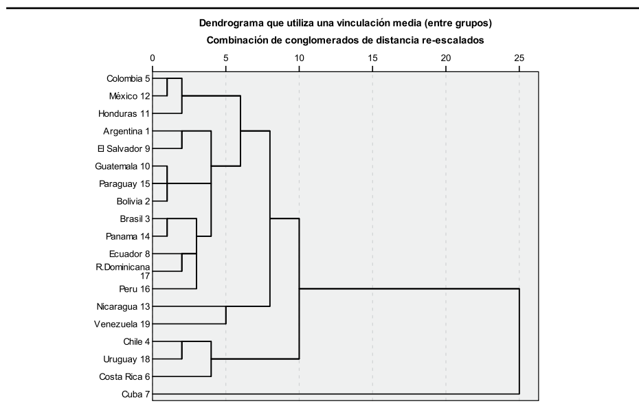
Gráfico 1 Dendograma de combinación de conglomerados
